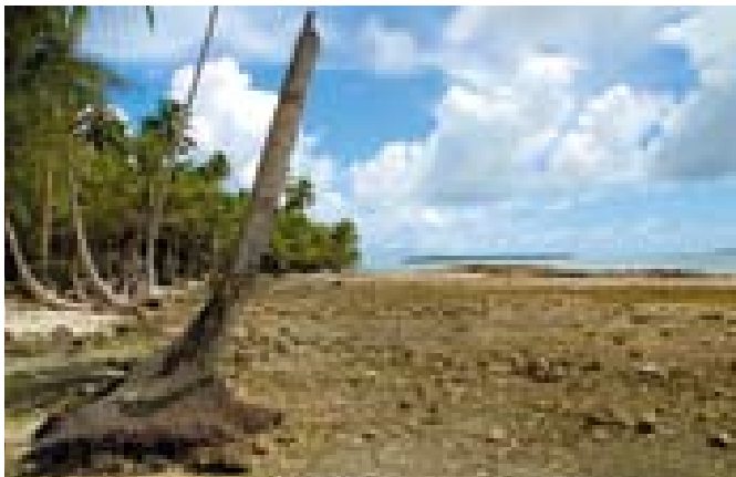
Erozija atola je posledica višanja morske gladine.
